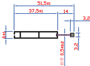
Half Panel 小叶片
