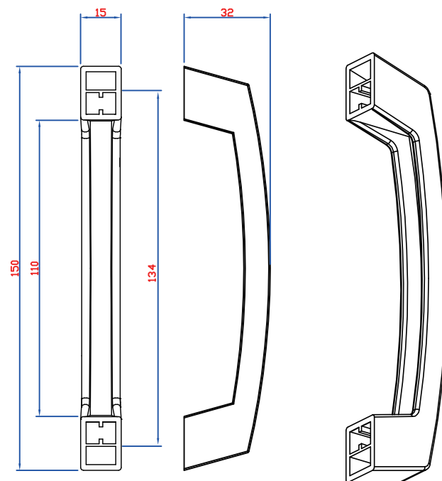
F1 Plastic Handle 2PCS In Accessories Bag 塑料把手 * 2件 用途:五金包
