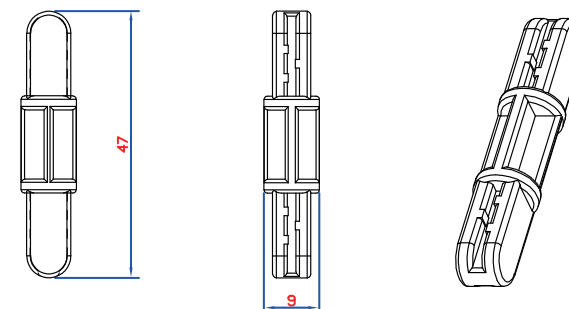
F2 Bolt 2PCS In Accessories Bag 插销 * 2件 用途:五金包
